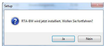
Abbildung 4: Sicherheitsabfrage
