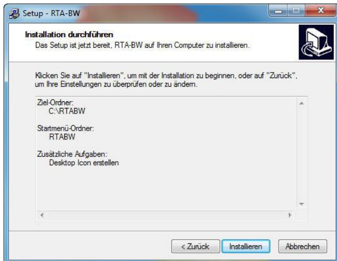
Abbildung 9: Installationsoptionen
