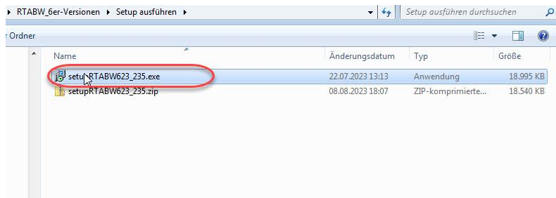
Abbildung 3: Setup-Datei entpacken
