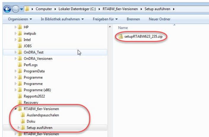
Abbildung 1: Download / Vorbereitungen
