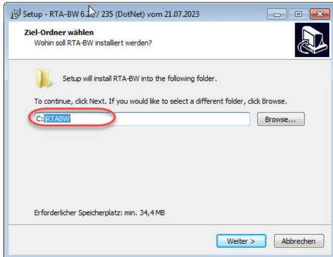
Abbildung 5: Installationsverzeichnis wählen
