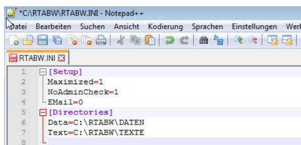
Abbildung 16: Konfigurationsdatei
