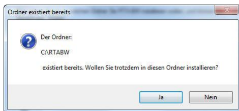
Abbildung 6: Warnhinweis
